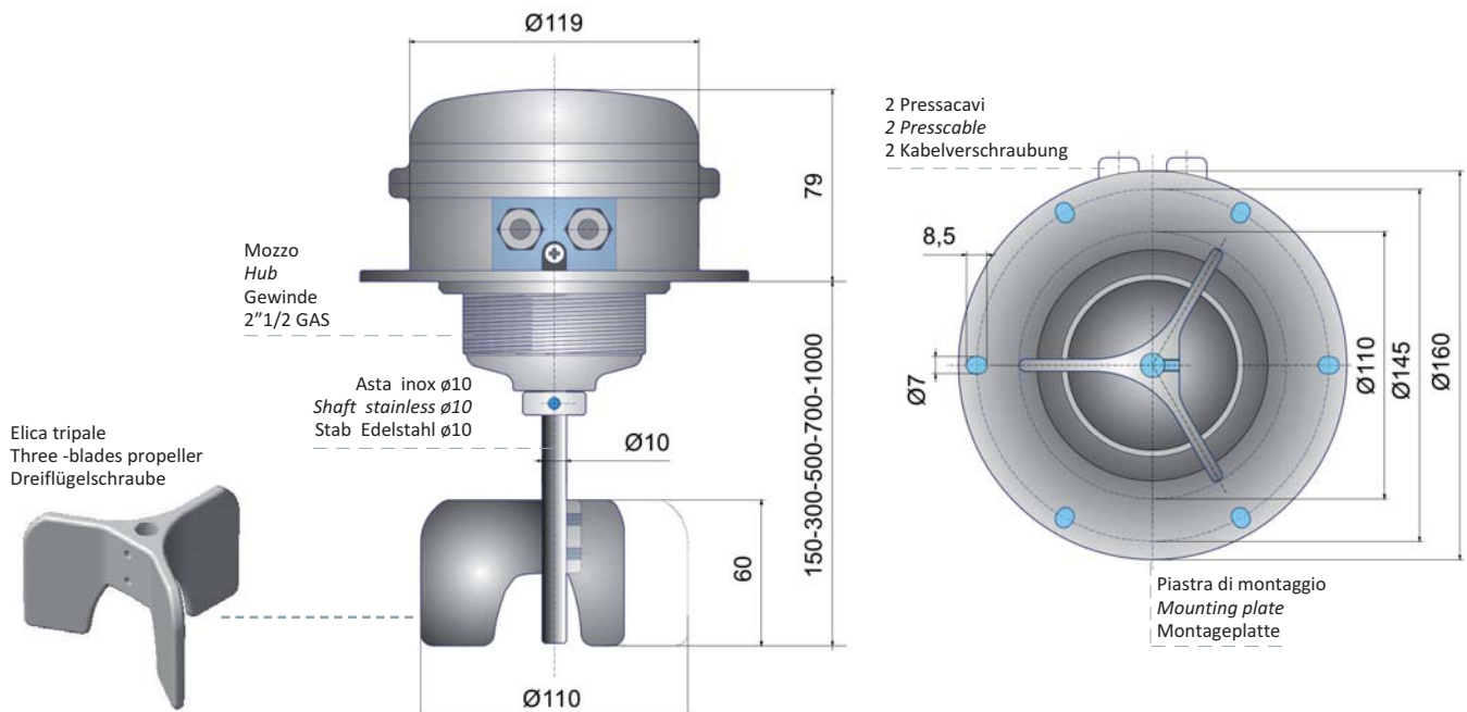
DIMENSIONI D'INGOMBRO - DIMENSIONS - ABMESSUNGEN
